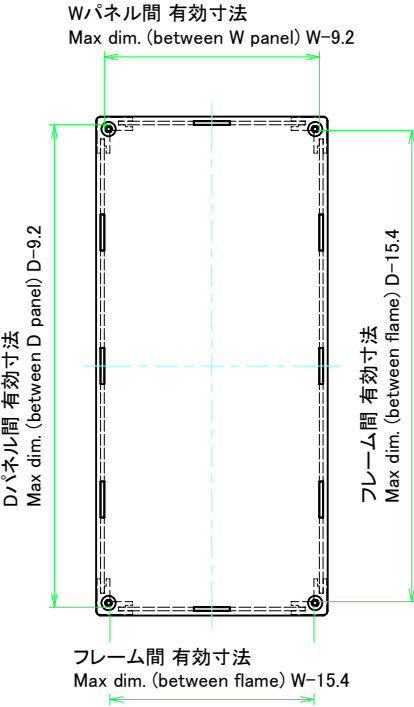
下カバー / Bottom cover
